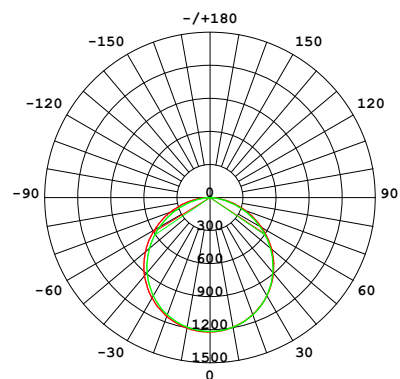
CURVA FOTOMETRICA
